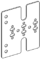
251-01-0086-00 尺寸 (長 X 寬 X 高) : 100mm x 2mm x 82mm 特殊用途扁頭安裝支架 以圓形和小型 U 型鎖孔 鎖固安裝於 Legrand MinkelsVaricon-M 機櫃中的 PDU。
