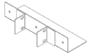
251-02-0023-00 尺寸 (長 X 寬 X 高) : 225mm x 68.7mm x 45.8mm 特殊用途雙柱安裝支架 用於鎖固淺口機架切換開關。
