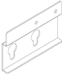
251-01-0032-00 尺寸 (長 X 寬 X 高) : 142mm x 12mm x 88mm U 型直立式並列安裝支架 以鑰匙孔形和圓形鎖孔 並列鎖固兩個 0U PDU。
