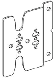
A0026-000001-000-1 尺寸 (長 X 寬 X 高) : 78.31mm x 9.9mm x 86.9mm 特殊用途安裝支架 以圓形和小型 U 型鎖孔 鎖固安裝於 Legrand Nexpand 機櫃中的 PDU。
