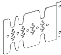
A0026-000002-000-1 尺寸 (長 X 寬 X 高) : 153.31mm x 9.9mm x 86.9mm 特殊用途安裝支架 以圓形和小型 U 型鎖孔 鎖固安裝於 Legrand Nexpand 機櫃中的 PDU。
